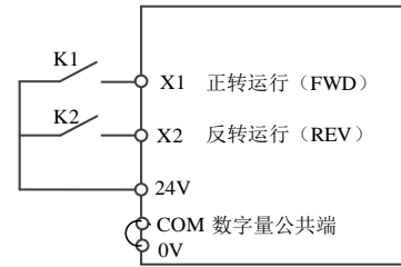
PNP型接法
