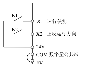
PNP型输入接法
