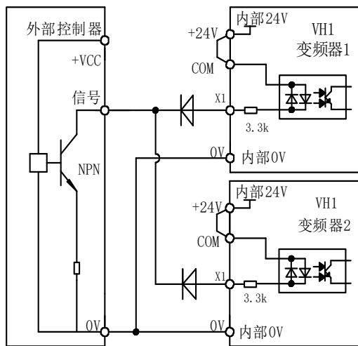
多台变频器使用变频器内部24V电源的漏型接线方法
