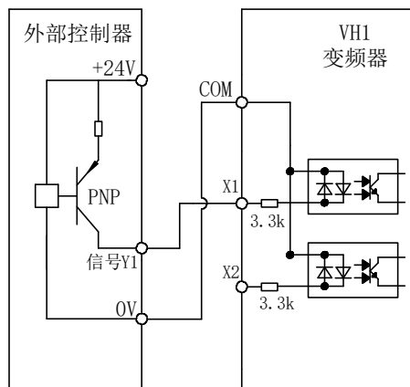
使用外部24V电源的源型接线方法
