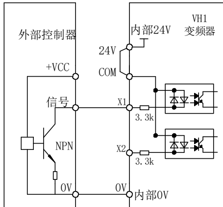
使用变频器内部24V电源的漏型接线方法
